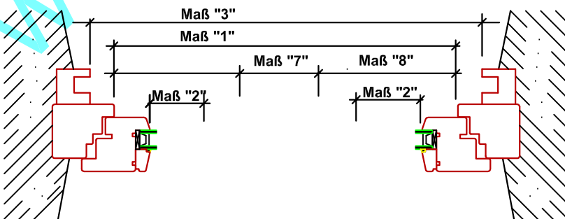
Fenster in der Breite mit Rolladen
